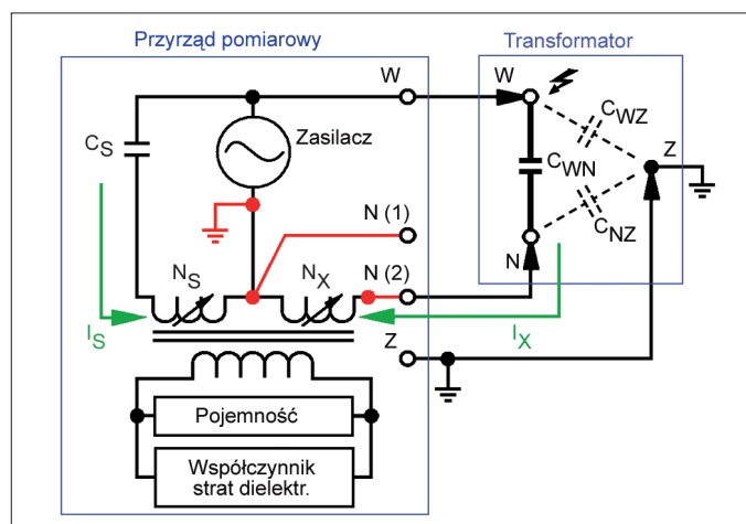
Rys. 5 Schemat układu pomiarowego w trybie pracy UST (pomiar między uzwojeniami)
