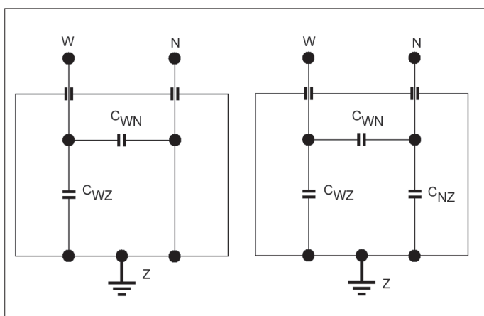
Rys. 1 Dwu- i trójbiegunowy układ zastępczy
