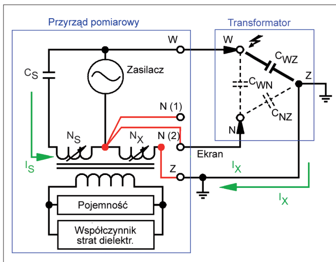
Rys. 6 Schemat układu pomiarowego w trybie pracy GST (pomiar między uzwojeniem i ziemią przy pozostałych uzwojeniach podłączonych do ekranu)
