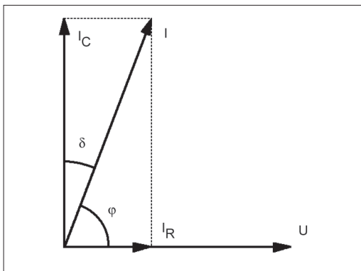
Rys. 2 Wykres wskazowy prądu i napięcia badanej izolacji
