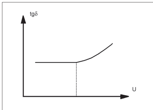
Rys. 3 Zależność współczynnika strat dielektrycznych od napięcia próby w obecności zjawiska jonizacji
