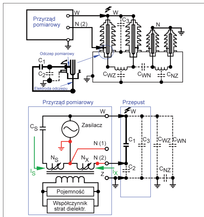
Rys. 7 Sposób podłączenia przyrządu pomiarowego podczas pomiaru przepustu transformatora oraz schemat układu pomiarowego w trybie pracy UST
