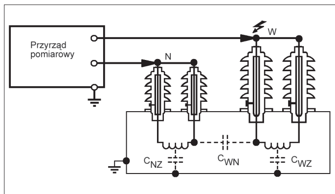
Rys. 4 Sposób podłączenia przyrządu pomiarowego do transformatora z dwoma uzwojeniami
